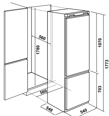
Logement d'encastrement Installation drawing
