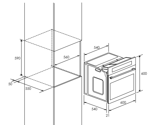
Logement d'encastrement Installation drawing
